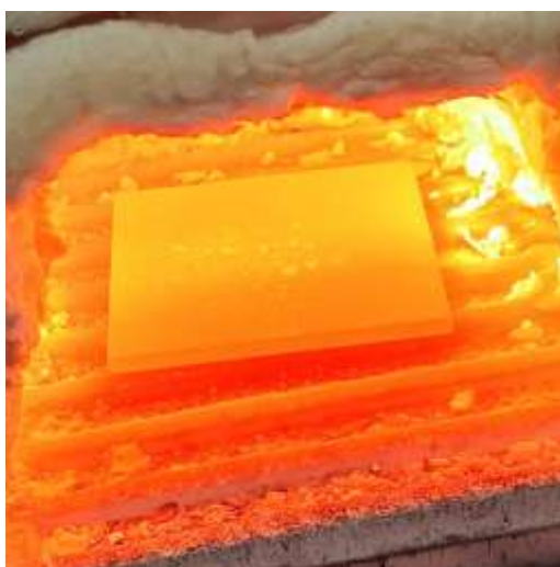
Ohřev ocelového podstavce v kovářské peci
