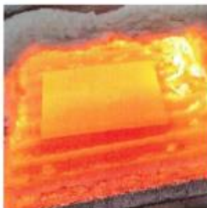
Dhřev ocelového podstavce v kovářské peci
